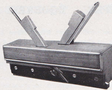
N° 38 BOUVET A JOINDRE 1 MORCEAU LANGUETTE FER
